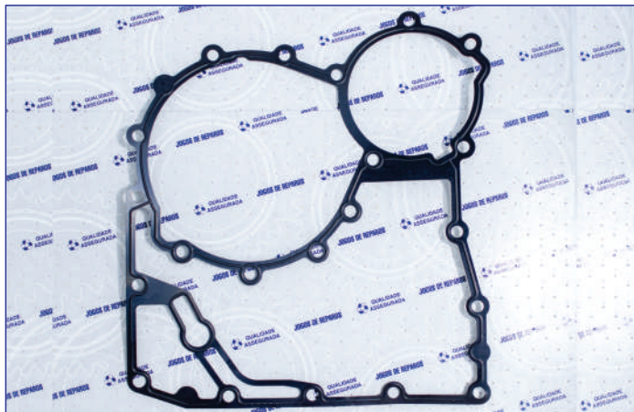
1766023 – JUNTA DO RETARDER GR 875 R, GRS 895 R, GR-GRS-GRSO 905 R, GRSO 925 R
