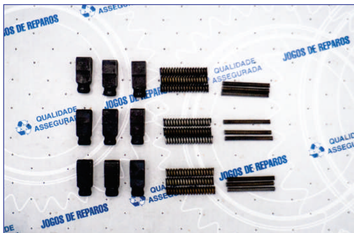
1250 198 400 – JOGO DE PRESSIONADOR S6-80, S6-90
