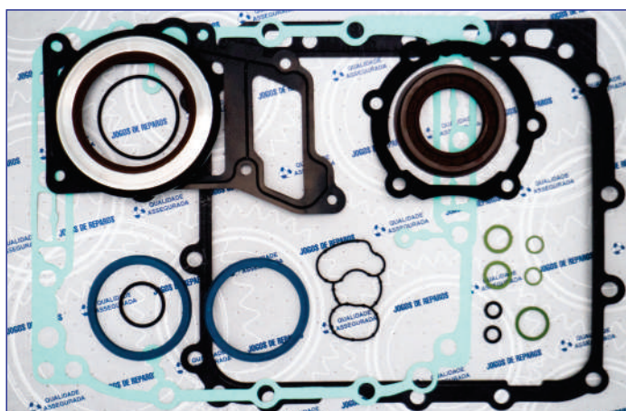
DP054 – JOGO DE REPARO COMPLETO I-SHIFT (METAL) AT 2412C, AT/ATO 2512C, AT/ATO 2612D, AT 2812C/D, ATO 3112C/D
