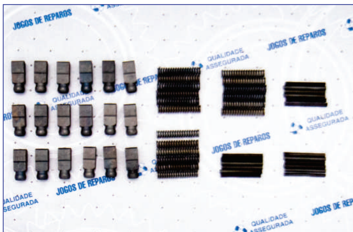
1295 198 402 – JOGO DE PRESSIONADOR 16S1300, 16S1600, 16S1900
