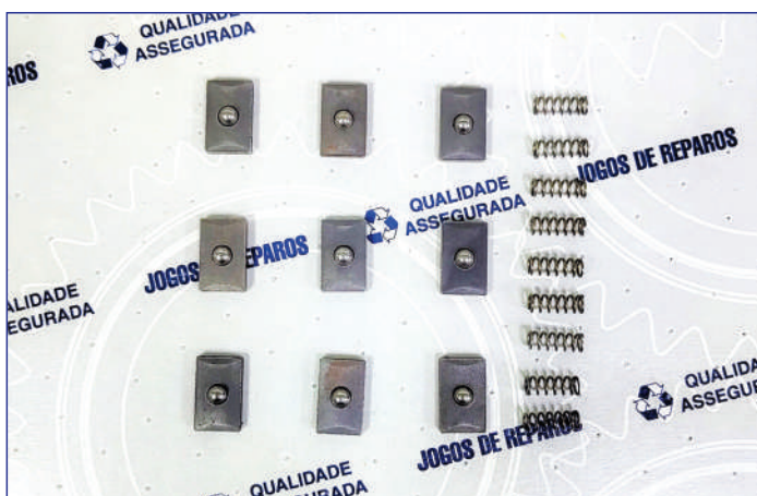
1307 198 412 – JOGO DE PRESSIONADOR S5-42, S5-420, 5S-580 BO/TO
