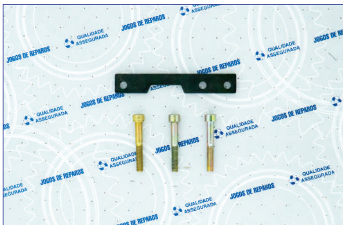
20845917 – BARRA DE APOIO FH 12 2001-2005, FM 9 2001-2005, FM 12 2001-2005
