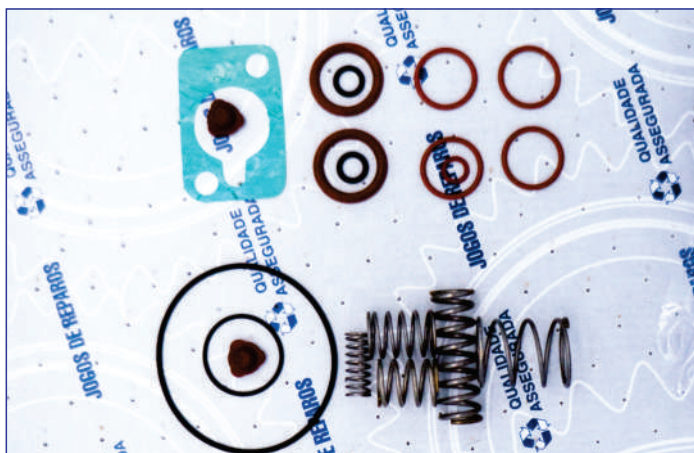
DP090 – JOGO DE REPARO VÁLVULA 5/2 VIAS 16S1300 - 16S1600 - 16S1650
