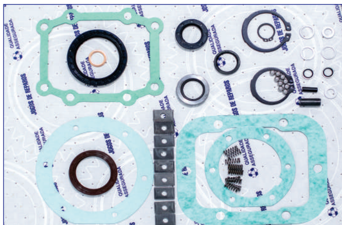
1307 298 810 – JOGO DE REPARO COMPLETO S5-420 8-150 E OD
