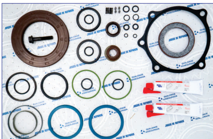
DP042 – JOGO DE REPARO COMPLETO VT2014/VT2214 COM RETENTOR 1652276 - 90X145X10
