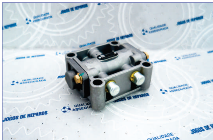
0501 396 633 – VÁLVULA DE 5/2 VIAS 16S1300 - 16S1600 - 16S1650
