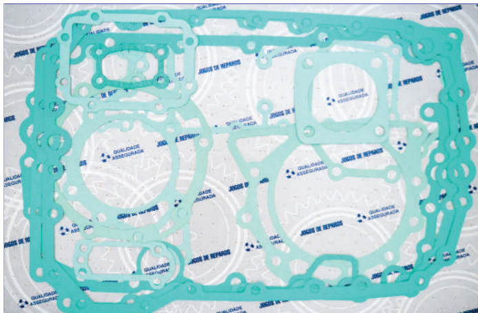
1295 298 891 – JOGO DE JUNTAS 8S-1350, 16S1300, 16S1600, 16S1650, 16S1900
