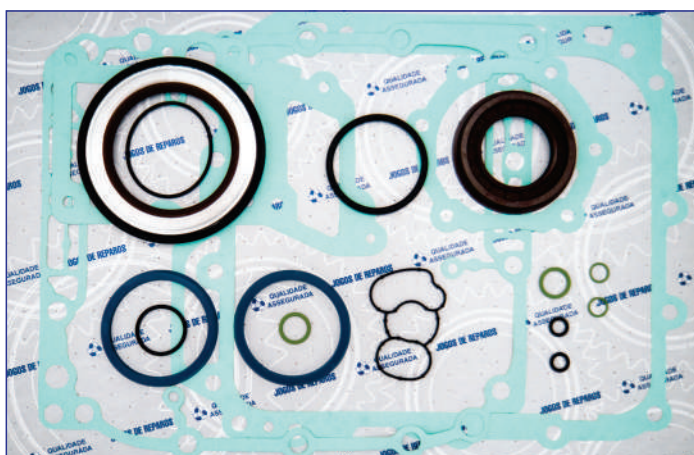
DP052 – JOGO DE REPARO COMPLETO I-SHIFT AT 2412C, AT/ATO 2512C, AT/ATO 2612D, AT 2812C/D, ATO 3112C/D
