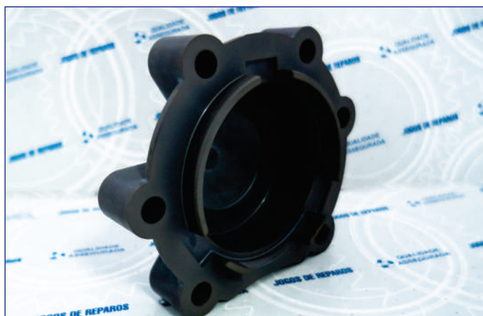
20483327 – TAMPA DO CILINDRO DA CAIXA FREIO AT 2412C/D, AT/ATO 2512C, AT/ATO 2612D, AT 2812C/D, ATO 3112C/D/E, ATO 3512D/E
