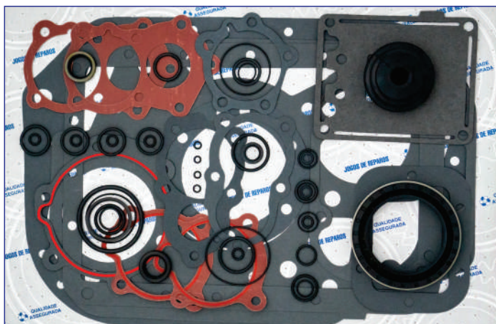
DP057 – JOGO DE REPARO COMPLETO FTS16112 / FTS20112
