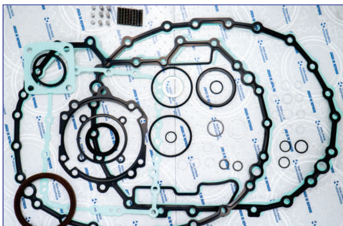
1328 298 017 – JOGO DE REPARO COMPLETO 12AS1930, 12AS2130, 12AS2530, 12AS2540, 16AS2230, 16AS2630, 16AS2631
